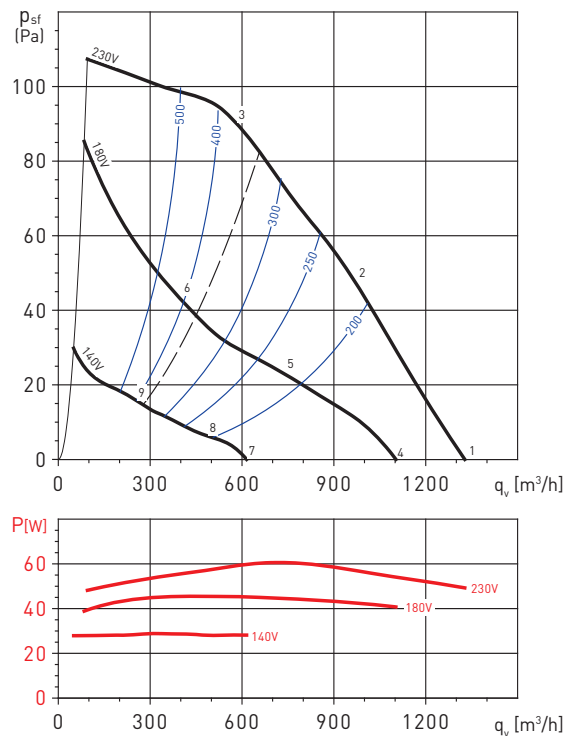
CTHB/6-225N
