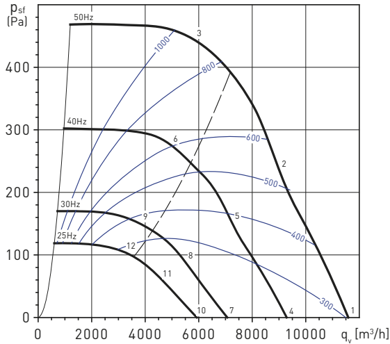
CTHT/6-500N
