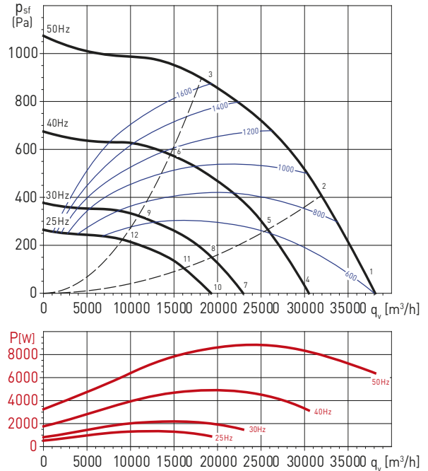
CTHT/6-710H 7,5 kW
