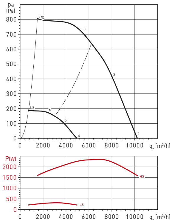
CTHT/4/8-450N
