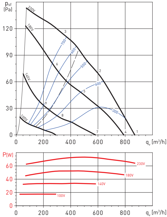
CTVB/4-180N
