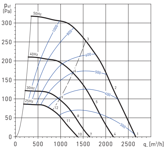
CTVT/4-250N
