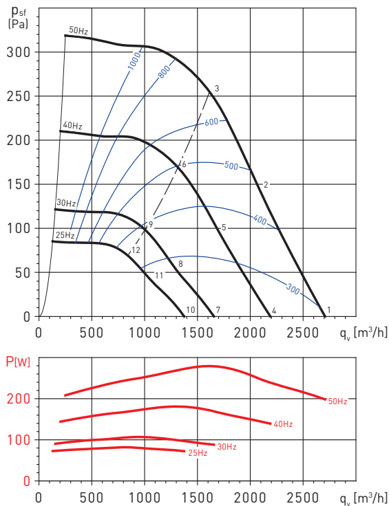
CTHT/4-250N
