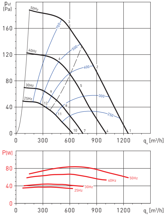
CTHT/4-200N
