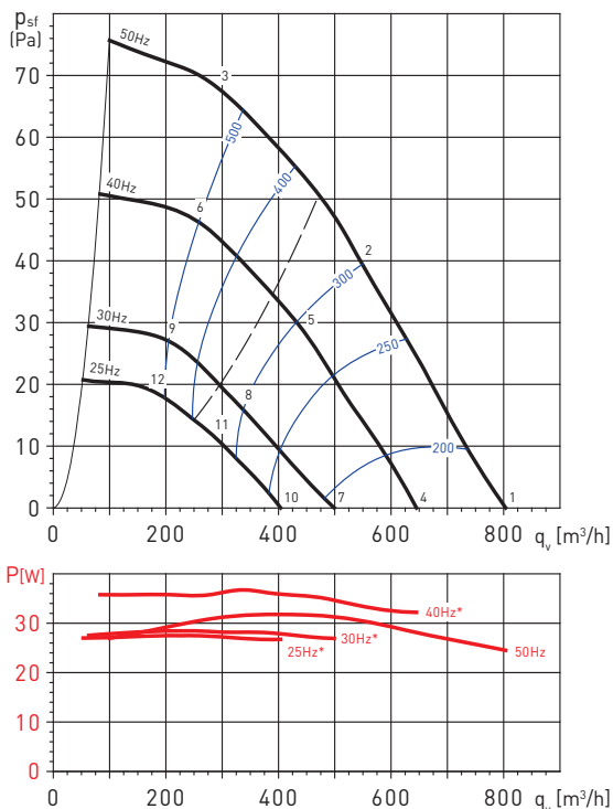
CTHT/6-200N
