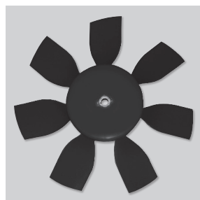
Hélice equilibrada dinámicamente , según norma ISO 1940, para reducir el ruido y evitar vibraciones.
