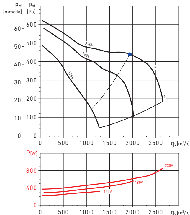
CVB/4-270/200 N 373W
