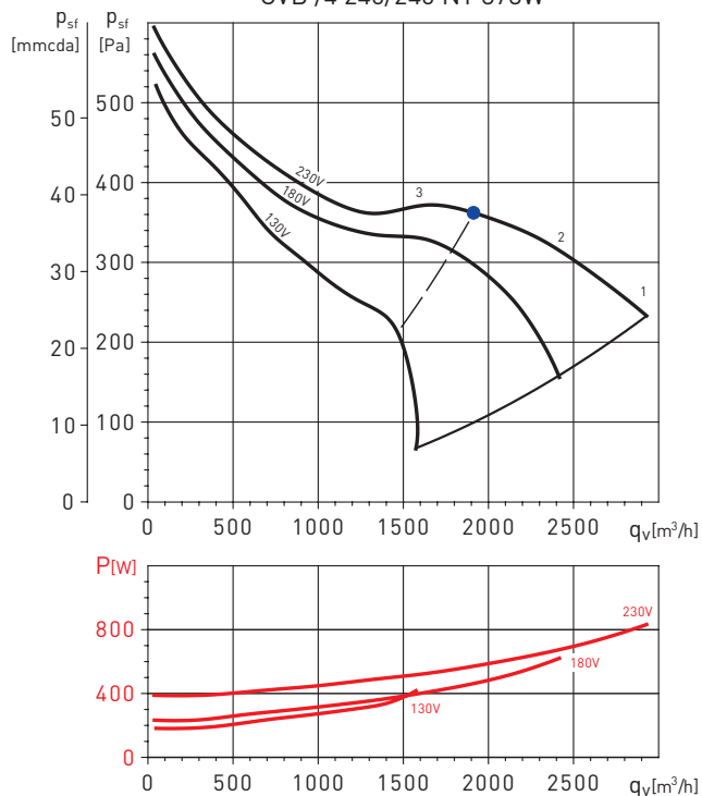
CVB /4 240/240 NT 373W
