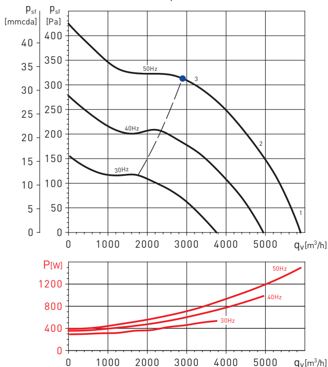
CVT-320/240 NT 1100W
