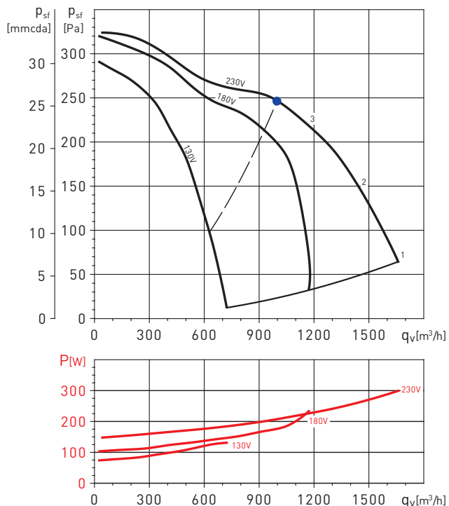
CVB /4 180/180 RE 147W
