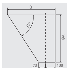
APC Viseras de aspiración o descarga Evitan la entrada de agua o cuerpos extraños en la instalación o en los ventiladores.
