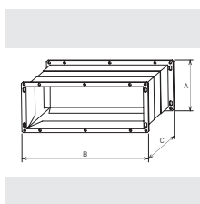
ACOP RECT F400 Acoplamiento elástico rectangular Para instalar en la descarga. Evitan la transmisión de vibraciones. Capacitados para trabajar en condiciones de 400°C/2h.
