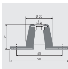
KSE Soportes antivibratorios Soportes antivibratorios de goma que permiten amortiguar las vibraciones y atenuar el nivel sonoro de la instalación. (1 KSE = 4 soportes en una bolsa)
