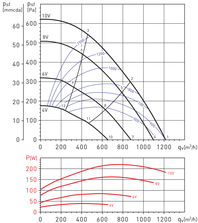
CAB-250 ECOWATT
