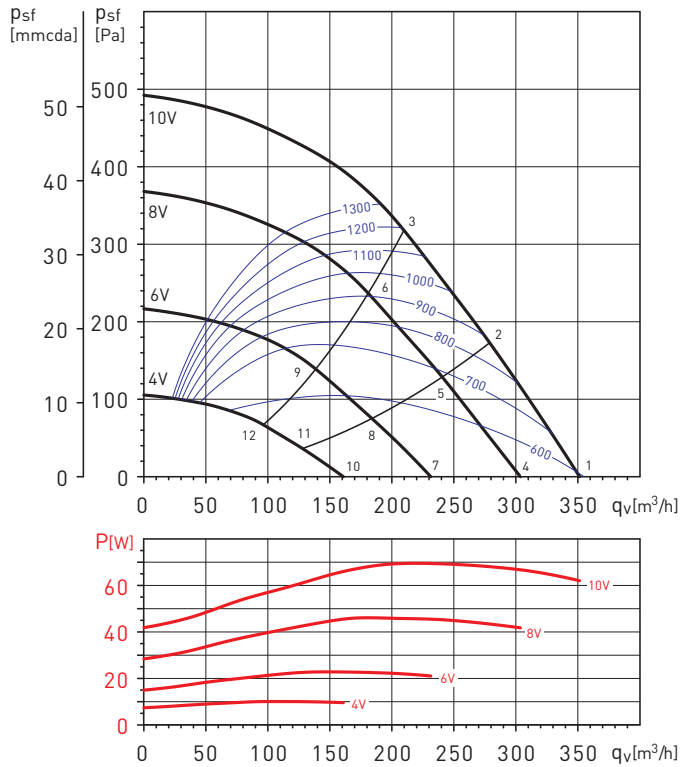
CAB-125 ECOWATT
