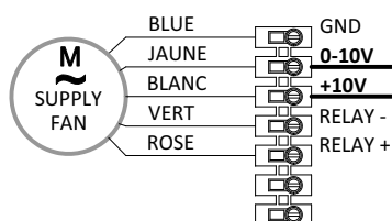
Ventilateur de soufflage
