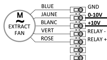
Ventilateur d'extraction
