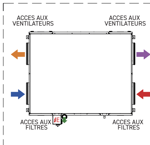
VUE DU DESSUS Ventilateur de soufflage sur le côté droit
