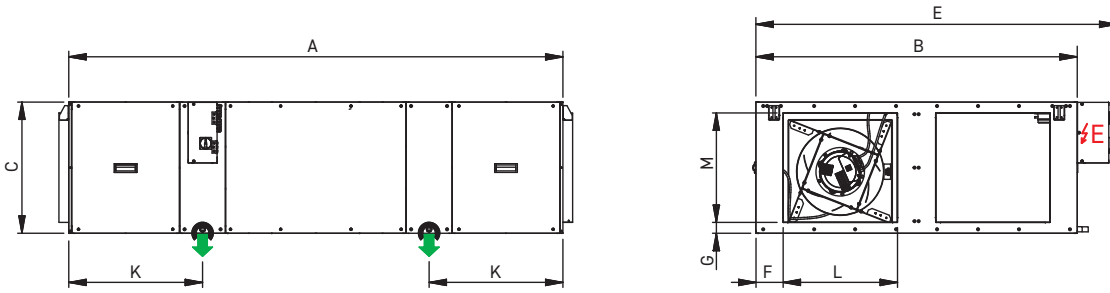
VUE DU DESSUS
