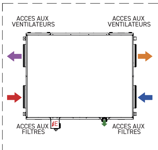
VUE DU DESSUS Ventilateur de soufflage sur le côté gauche (par défaut)
